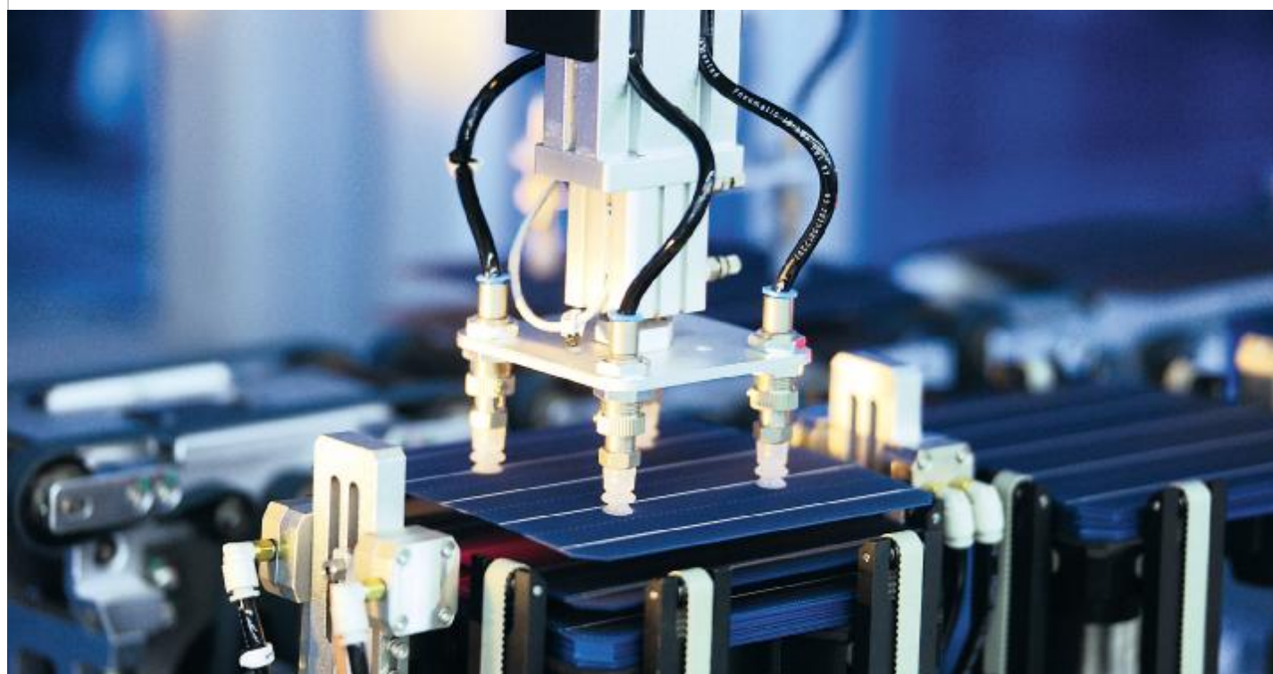
通威太阳能智能制造生产线
