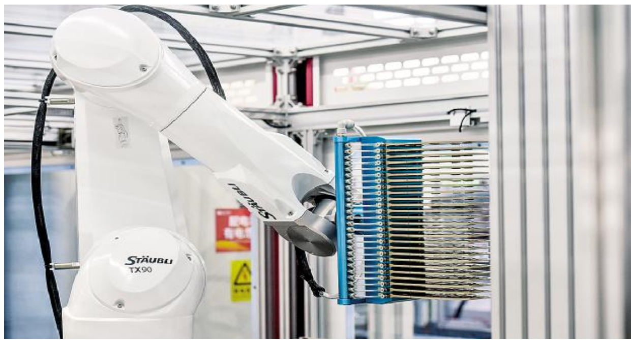
通威太阳能智能制造生产线机械臂
